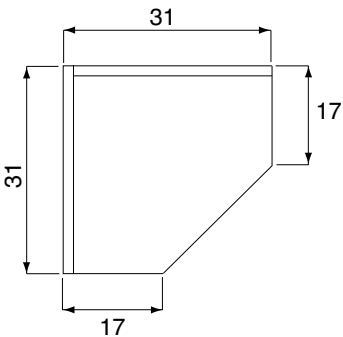
PENSILE TERMINALE a giorno tipo “A” Type “A” open END WALL UNIT
